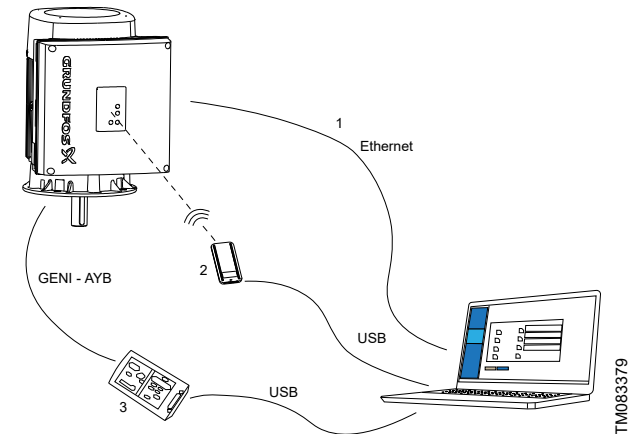
Grundfos GO Link setup
