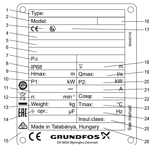
SEG and SEG AUTOADAPT nameplate
