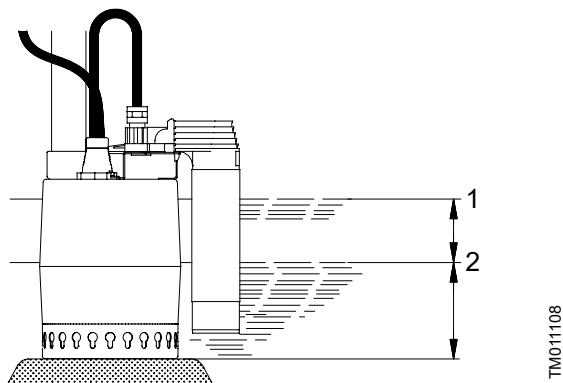
Start/stop levels for UNILIFT KP AV
