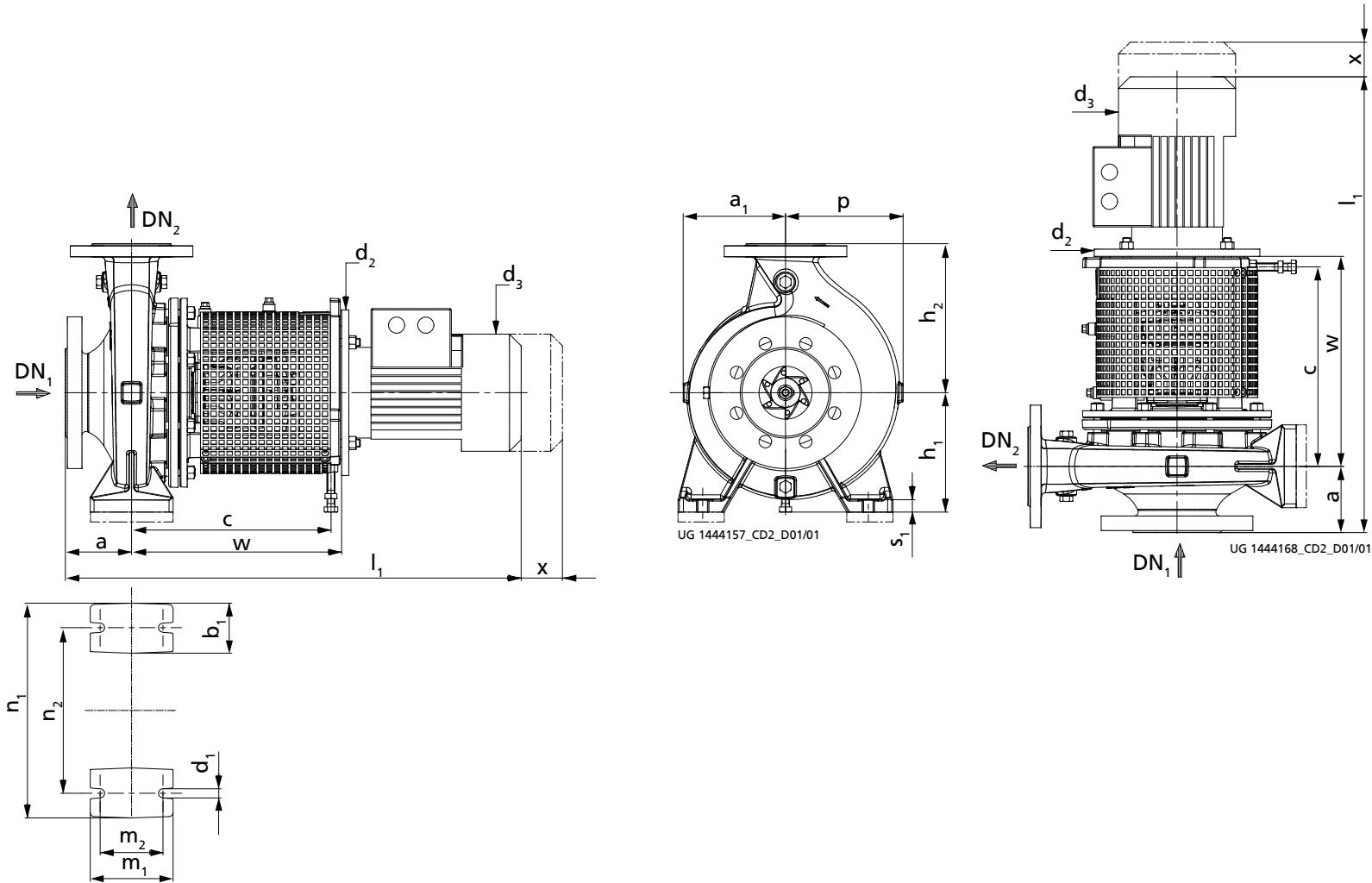
Fig. 3: Dimensions
