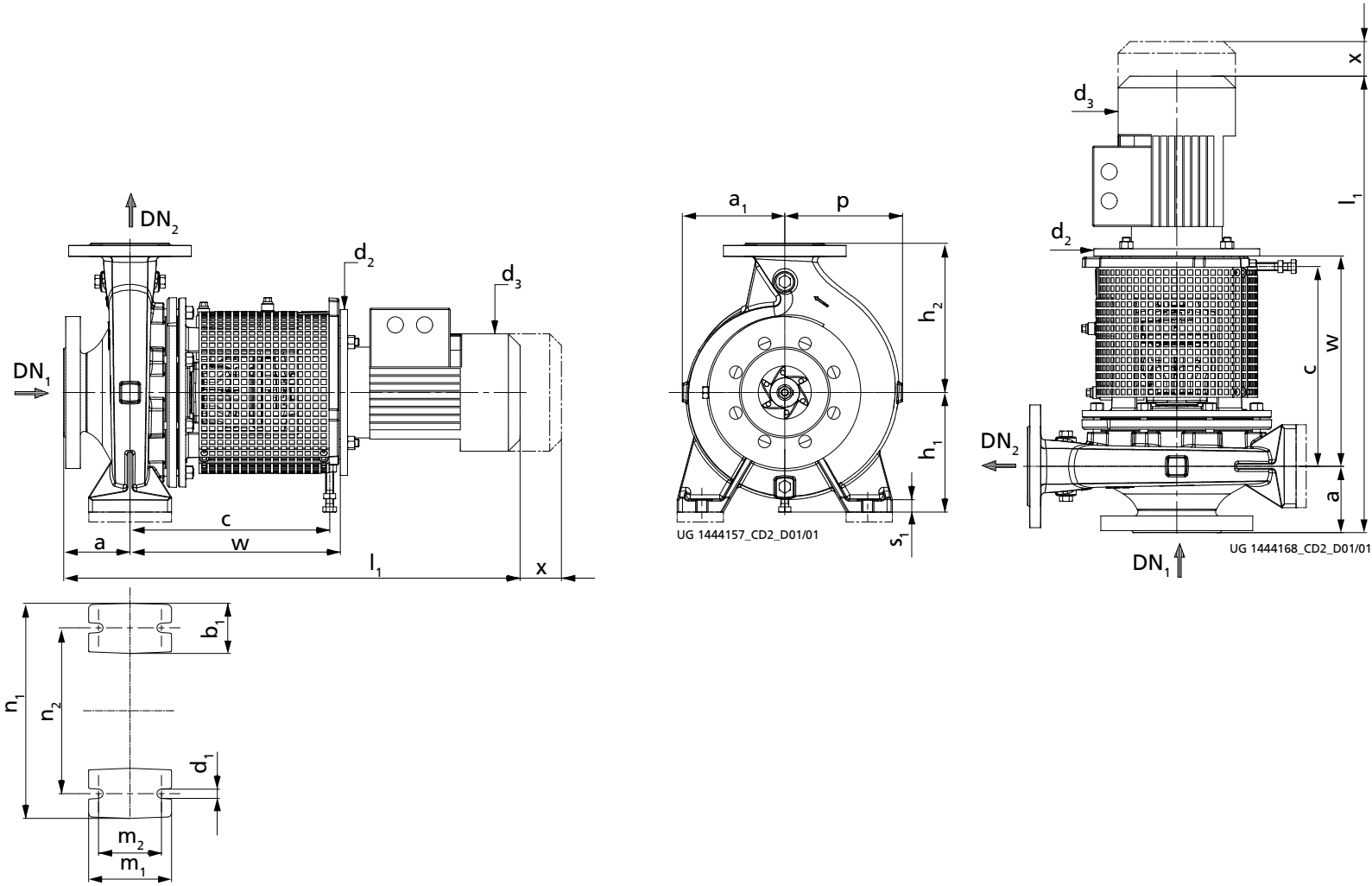
Fig. 2: Dimensions
