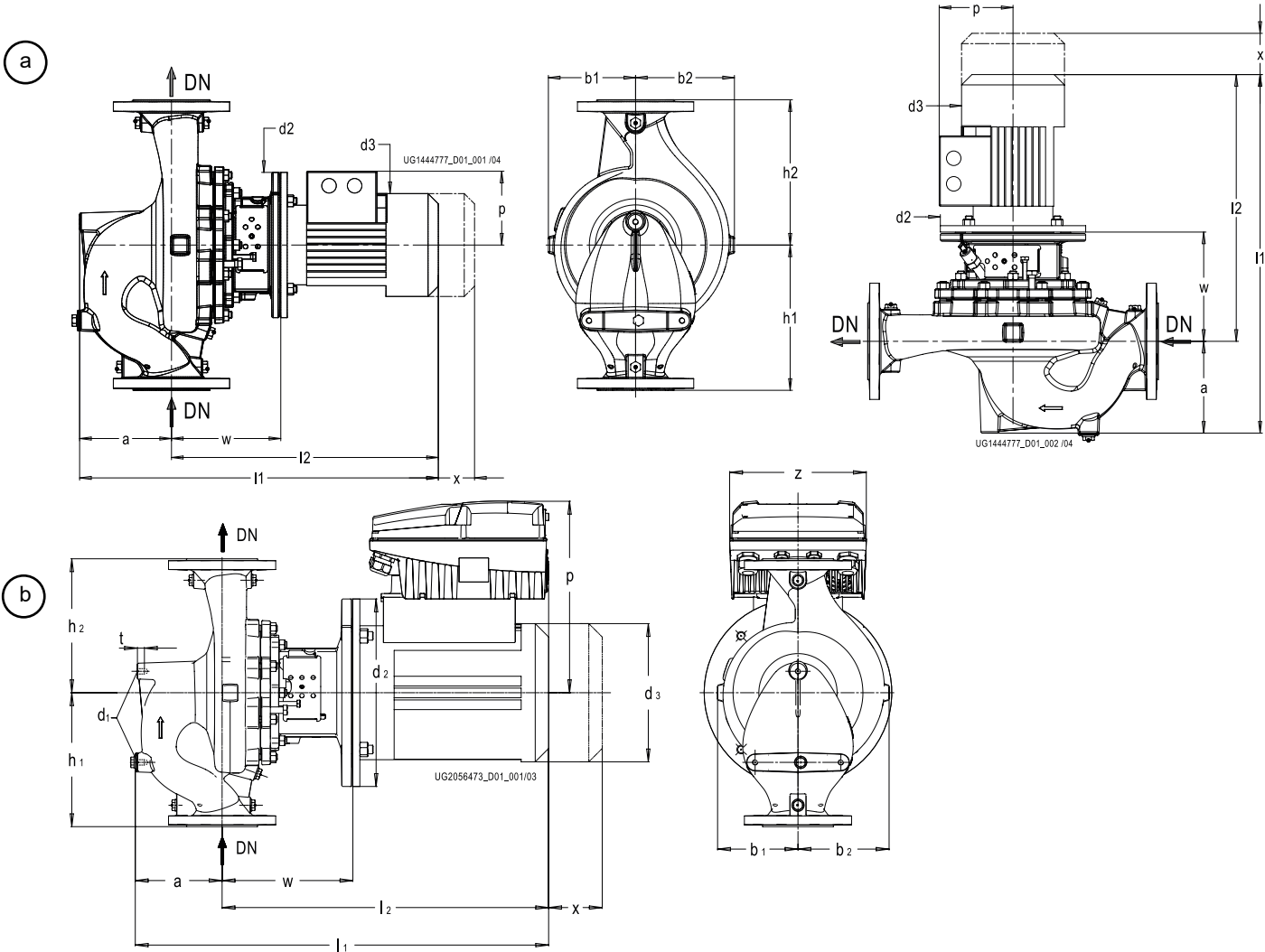
Fig. 4: Dimensions
