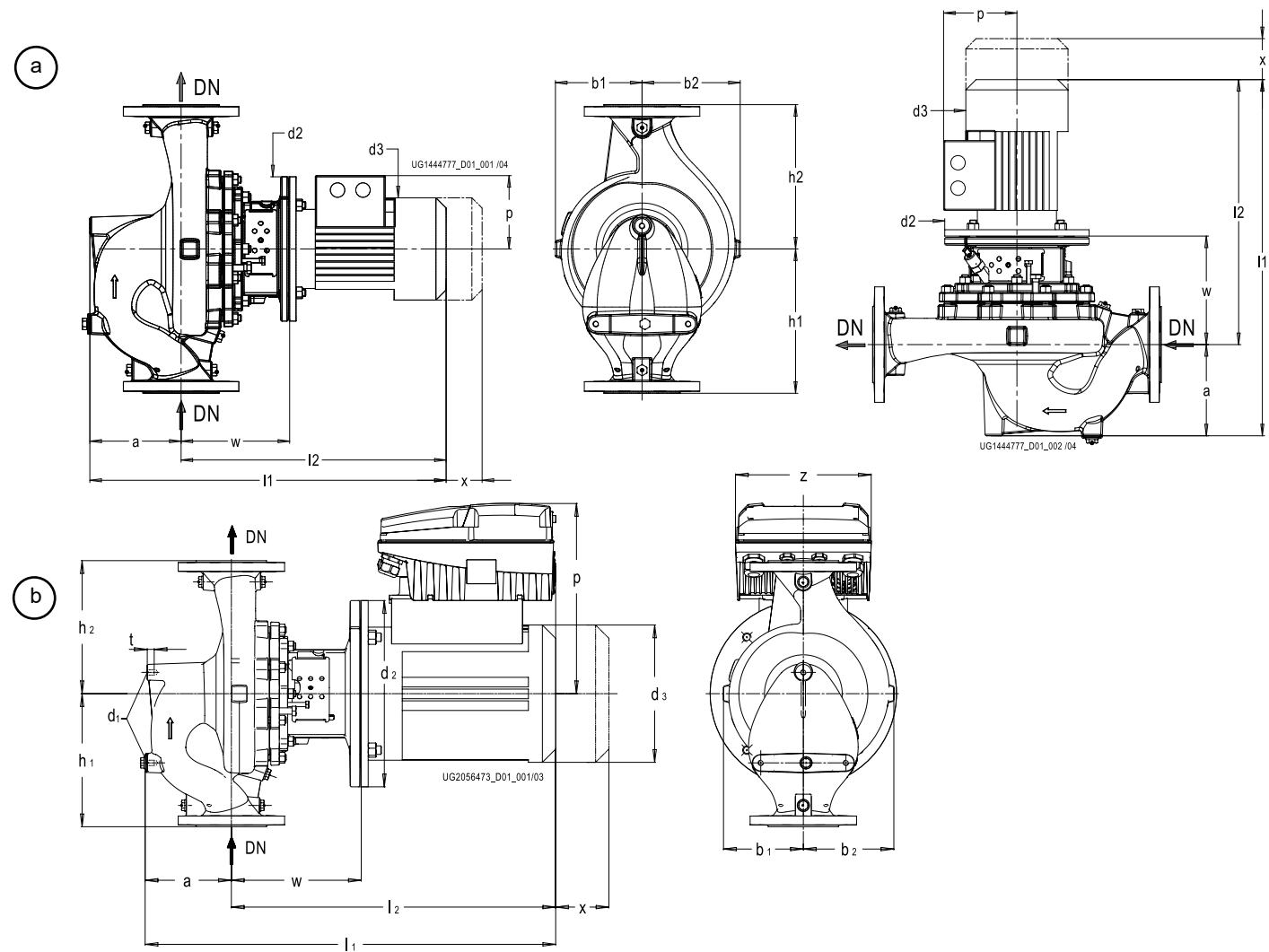
Fig. 2: Dimensions
