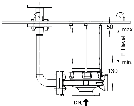
Fig. 4: Fill level
