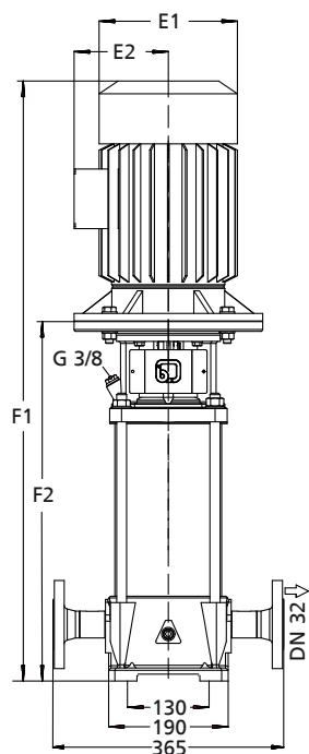
Movitec LHS dimensions
